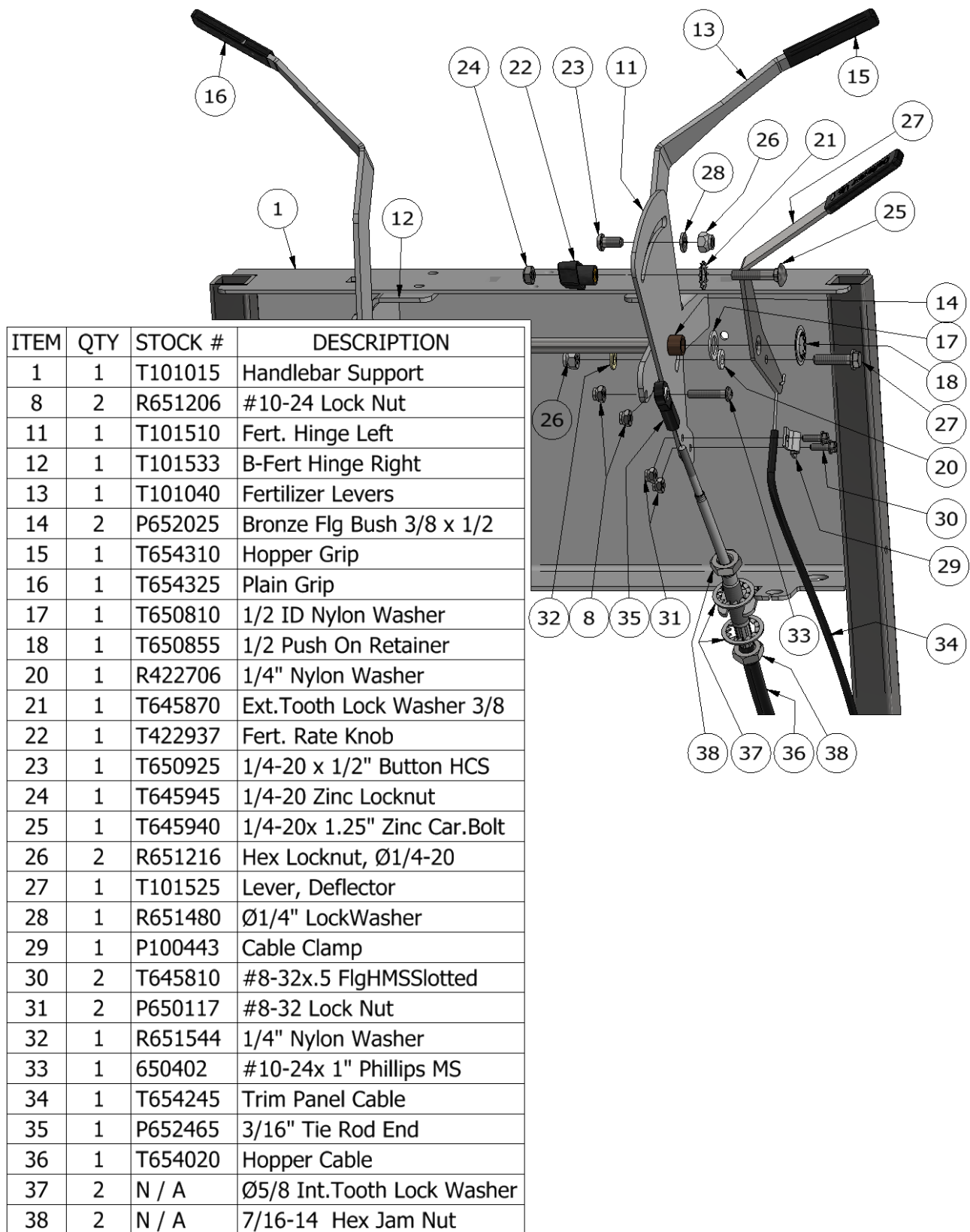
Fertilizer Levers Fig. 29.8
